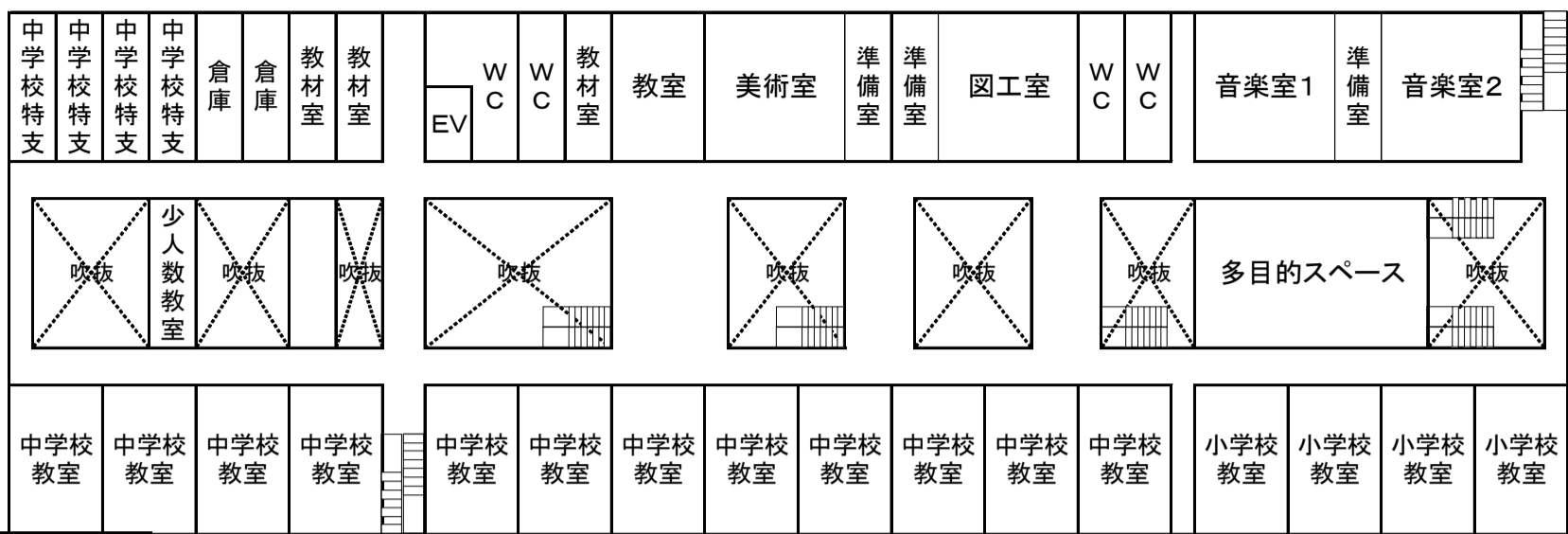
■3階平面図
